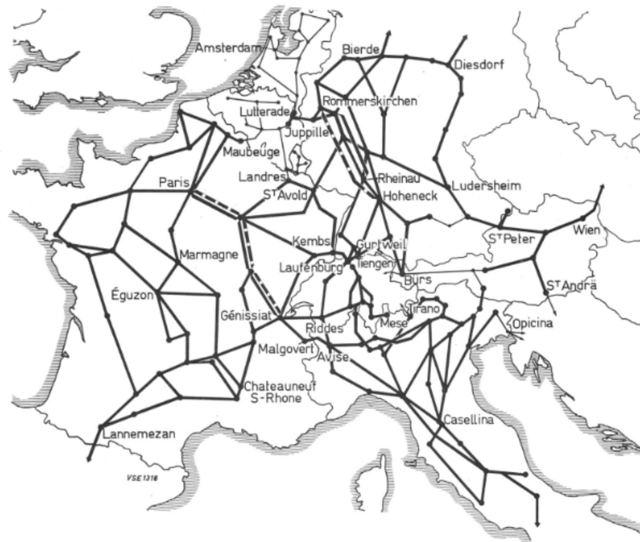
Fig. 2 220-kV-Netz der Länder der UCPTE — 220-kV-Leitungen
